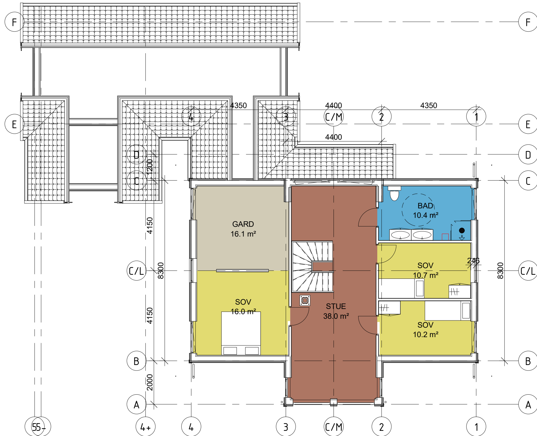
Plan 02 Copy 1 1 : 100
